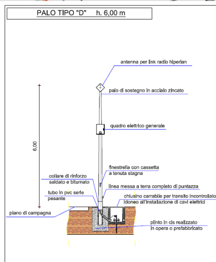
Particolare Costruttivo Palo diritto
