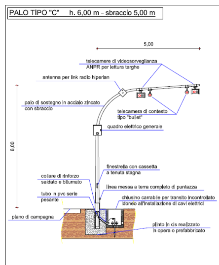
Particolare Costruttivo Palo a Sbraccio
