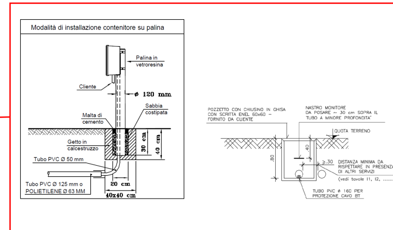
Predisposizione per nuovo contatore ENEL
